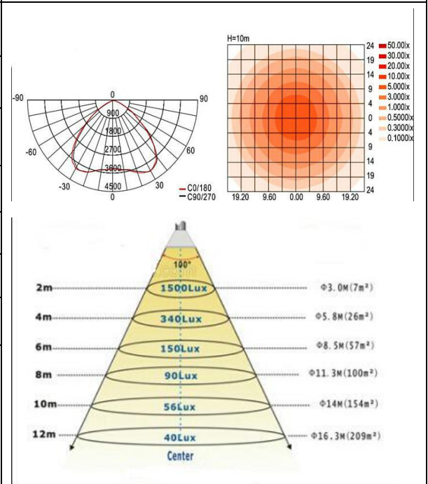
配光曲線圖
